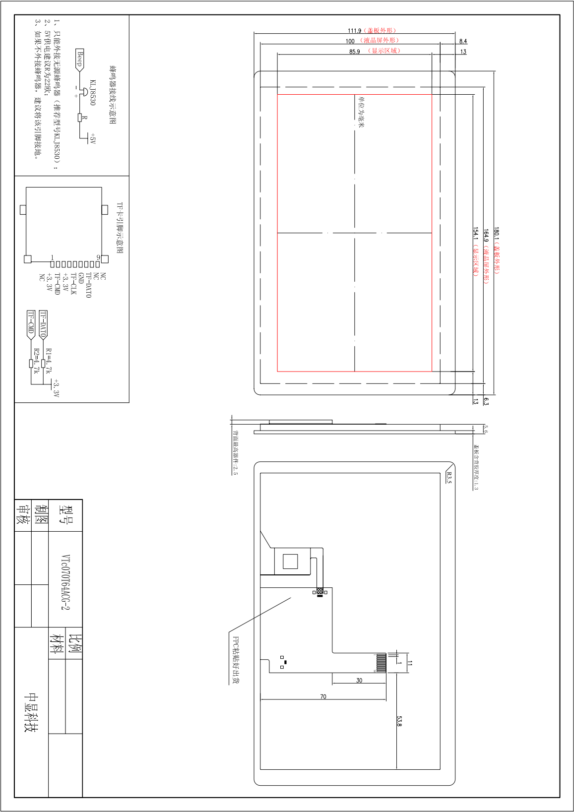
图 5 VTc070T64ACG-2 尺寸图
